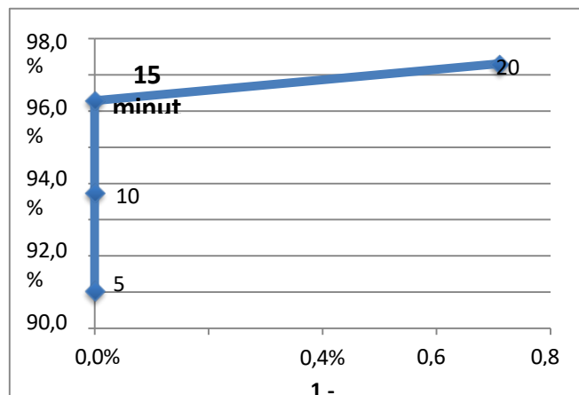
Figura 3. Curva ROC.
